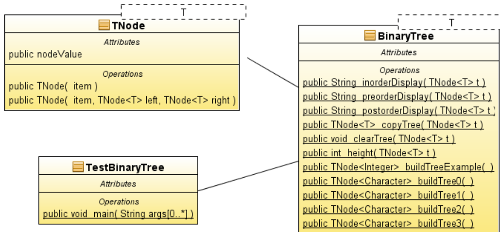
Gambar 6. Class Diagram dari praktikum Binary Tree
