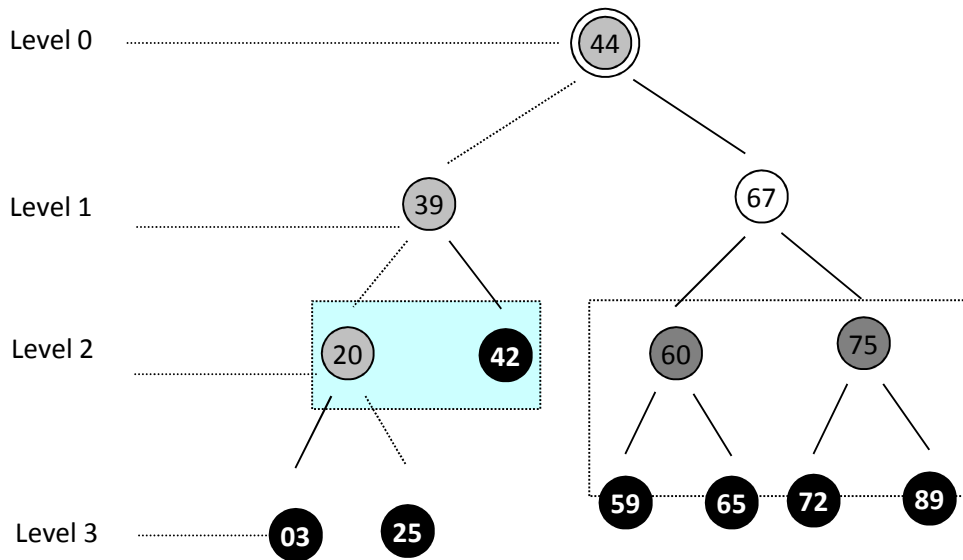
Gambar 16.1 Pohon Biner ( Binary Tree ) dengan kedalaman 3
